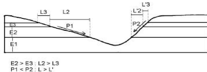
Fig.21 : Coupe
