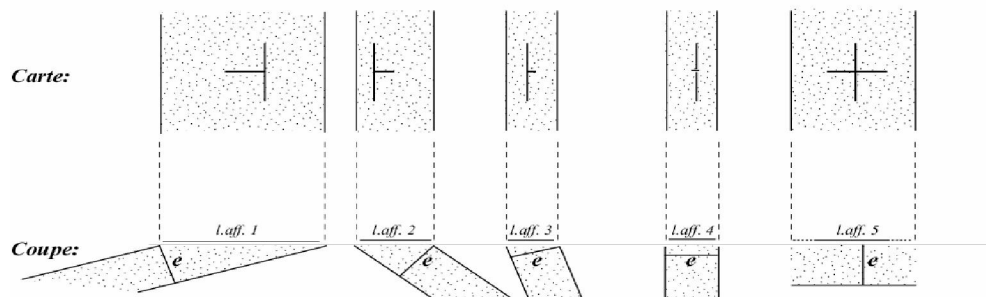
Fig. 22 : Relation entre la largeur d'affleurement, le pendage et l'épaisseur d'une couche
