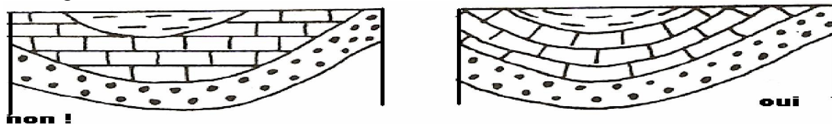
Fig. 1: Disposition des figurés dans des couches déformées
